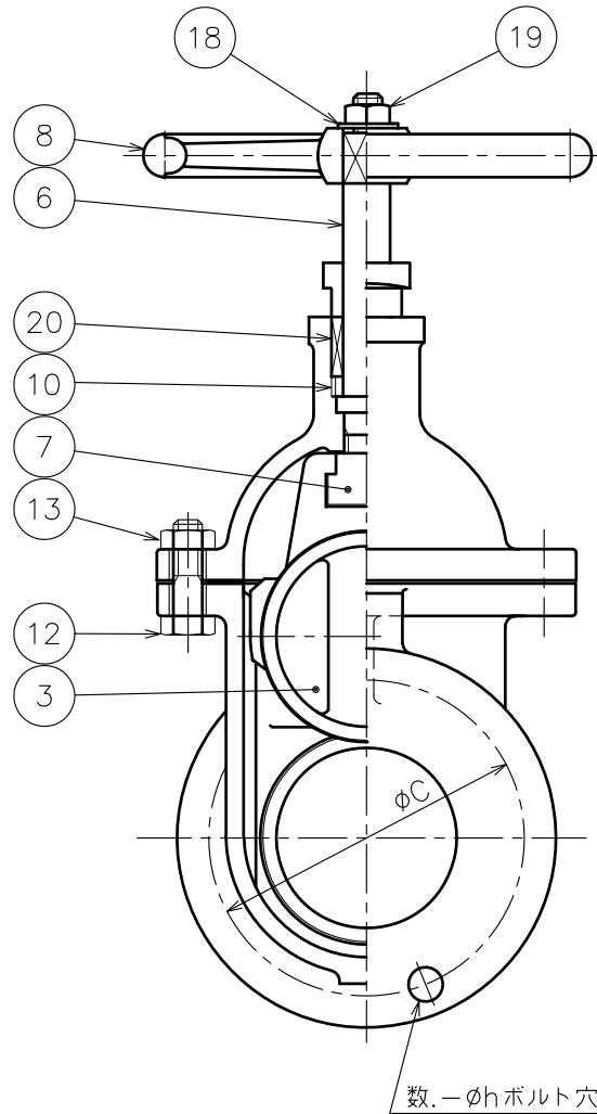
△ 単位：mm
